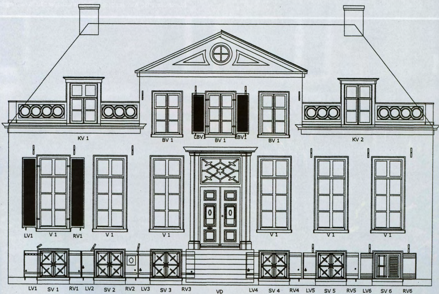
De bouwtekening die Pien Spijkers heeft vervaardigd van Vreeden Hoef' vormt, samen met onder meer een uitgebreide serie foto's, de basis voor Gerards' bouwproject'.
